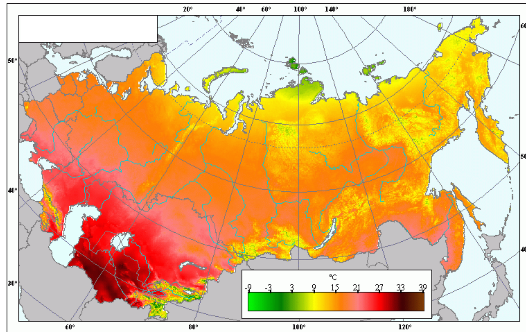
Средняя температура воздуха. Июль
