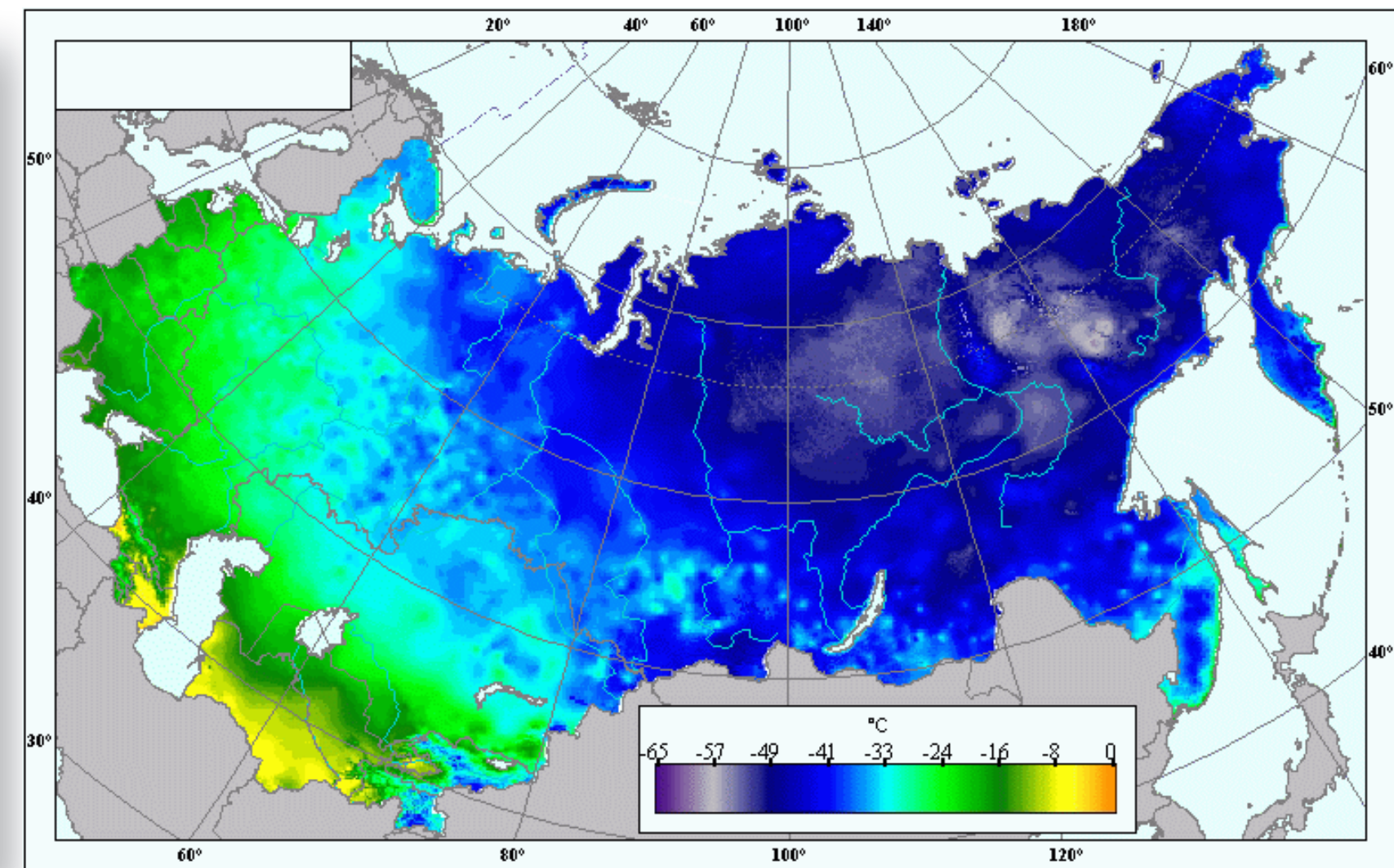
Средняя температура воздуха. Январь
